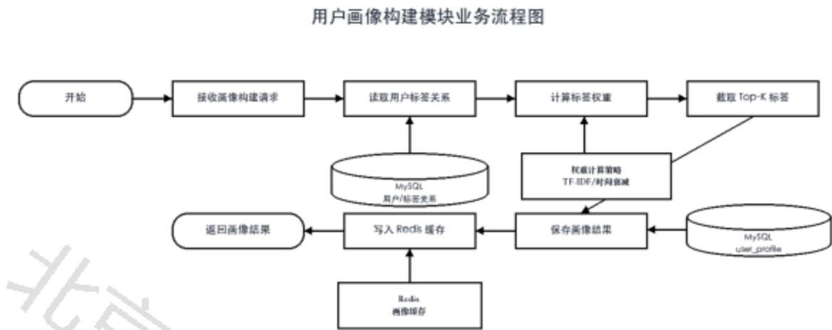
图 5-1 用户画像构建模块业务流程图
