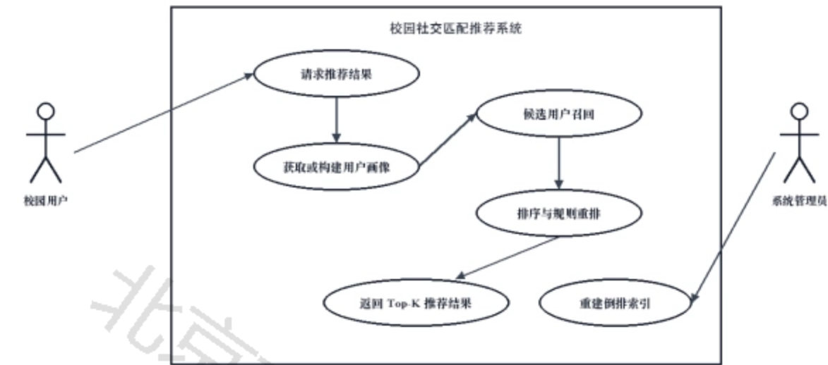
图 3-2 画像构建与推荐生成用例图
