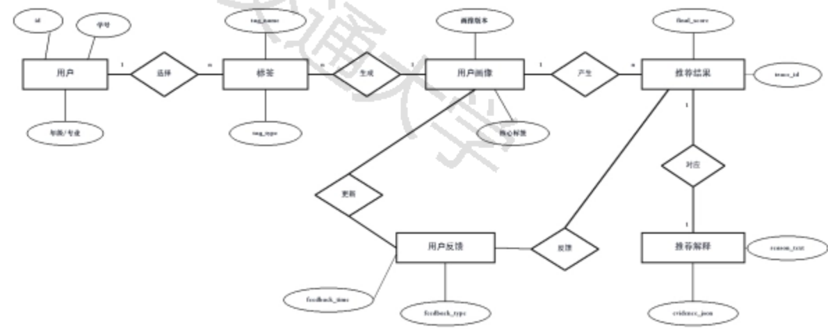
图 4-4 数据存储 ER 图
