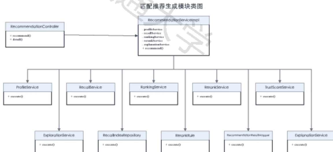
图 5-6 匹配推荐生成模块类图
